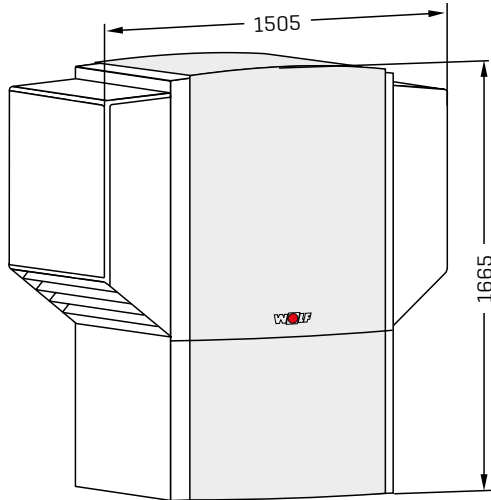
BWL-1-A - Außenaufstellung
